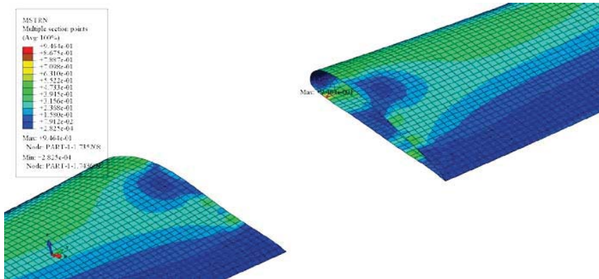
圖 19 破壞指標最高值發生處(第三次優化 MSTRN=0.9464)
