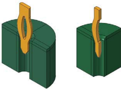
(a) 簡化模型 (a) 二分之一對稱模型 (b) 簡化模型 (b) 四分之一對稱模型
