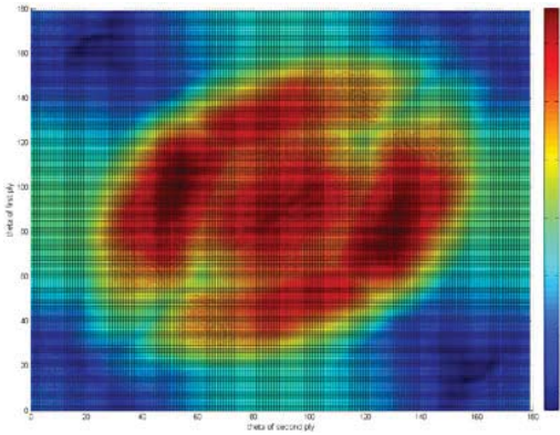
圖 15 長板長邊固定之等高線圖
