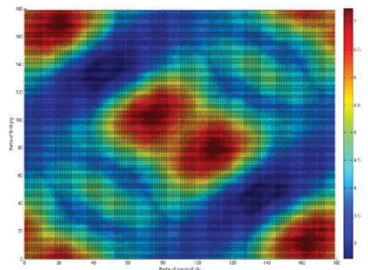
圖 18 方板四邊固定之等高線圖 (僅兩層疊層)
