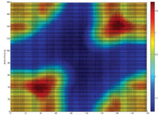
圖 16 方板單方向固定之等高線圖
