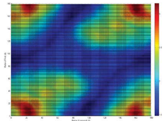
圖 17 方板四邊固定之等高線圖
