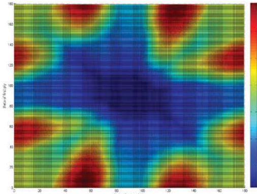
圖 13 長板短邊固定之等高線圖
