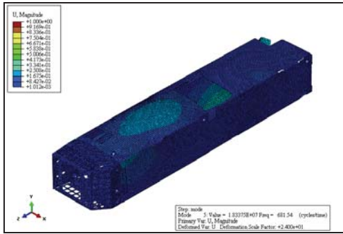
圖 13 第五模態 (681Hz)
