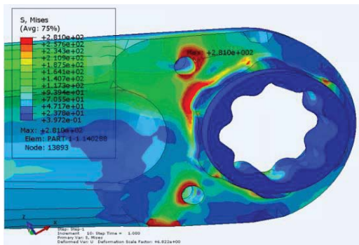
圖 17 改良設計的曲柄等效應力分布
