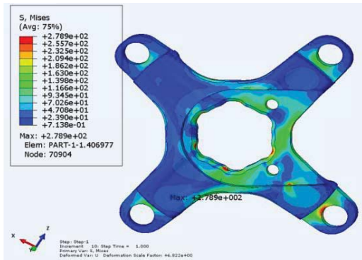
圖 16 改良設計的心盤等效應力分布
