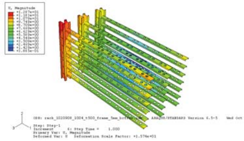
圖 21、模型二+BC2.2.3，溫昇 400 度，最大變形
