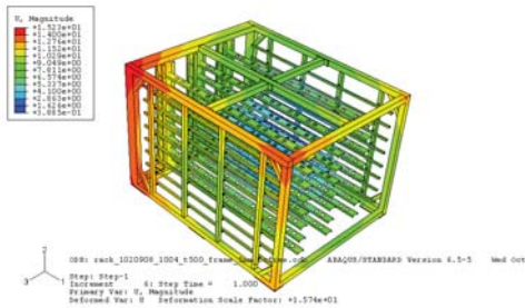
圖 18、模型二+BC2.2.3，溫昇 500 度，最大變形
