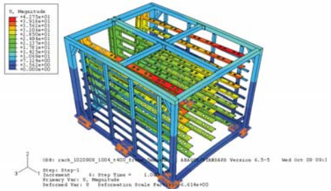
圖 13、溫昇 400 度，最大變形
