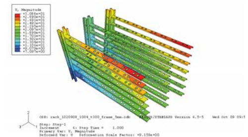
圖 16、溫昇 300 度，最大變形
