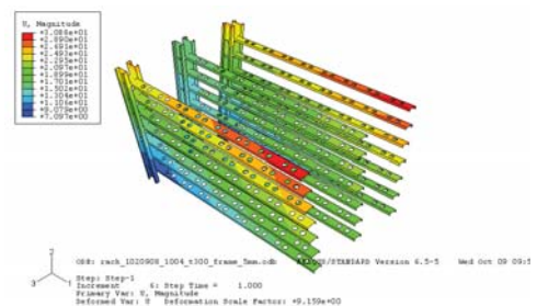
圖 16、溫昇 300 度，最大變形
