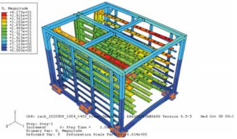
圖 13、溫昇 400 度，最大變形
