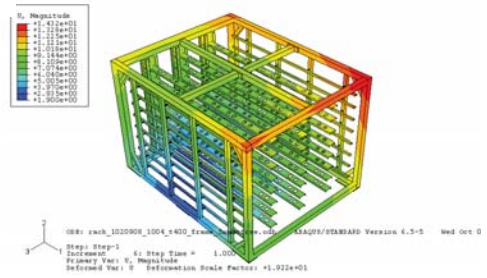
圖 19、模型二+BC2.2.3，溫昇 500 度，最大變形
