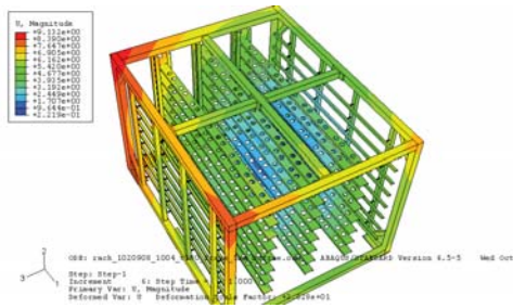
圖 22、模型二+ BC2.2.3，溫昇 300 度，最大變形
