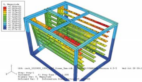
圖 10、轉角處補強取消 (模型二)
