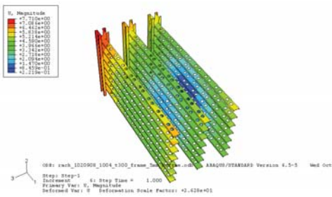
圖 23、模型二+ BC2.2.3，溫昇 300 度，最大變形
