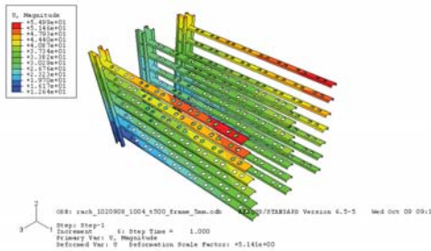
圖 12、溫昇 500 度，最大變形
