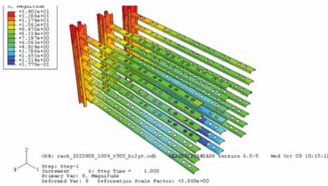
圖 17、模型一+BC2.2.2，溫昇 500 度，最大變形
