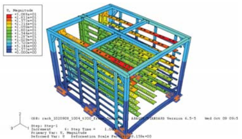
圖 15、溫昇 300 度，最大變形
