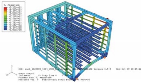
圖 17、模型一+BC2.2.2，溫昇 500 度，最大變形
