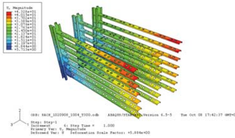
圖 9、溫昇 300 度，最大變形
