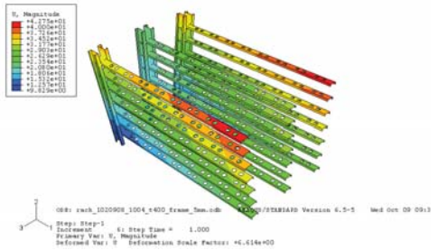
圖 14、溫昇 400 度，最大變形
