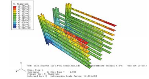
圖 14、溫昇 400 度，最大變形
