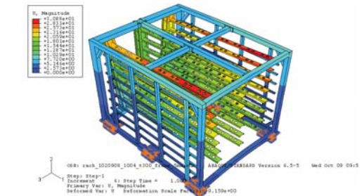
圖 15、溫昇 300 度，最大變形
