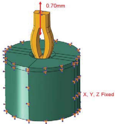
圖 4 邊界條件設定
