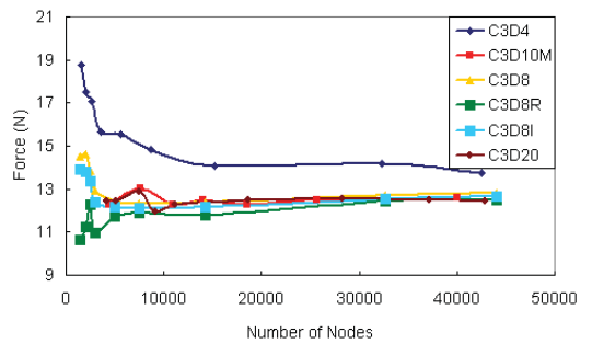
圖 7 不同元素之插入力比較
