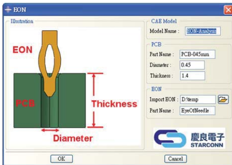
圖 10 RSG 客製化模組之示意圖
