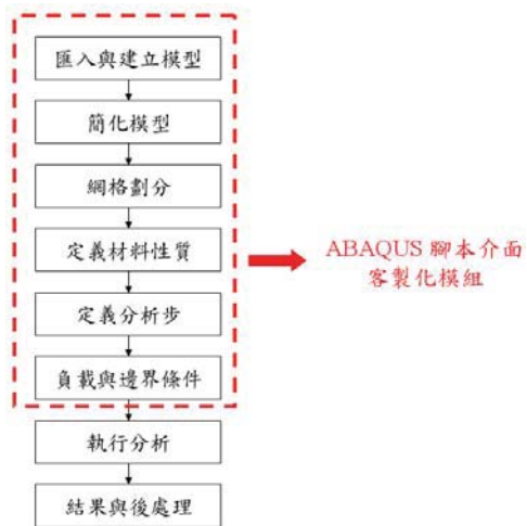
圖 9 分析步驟寫入客製化模組之示意圖
