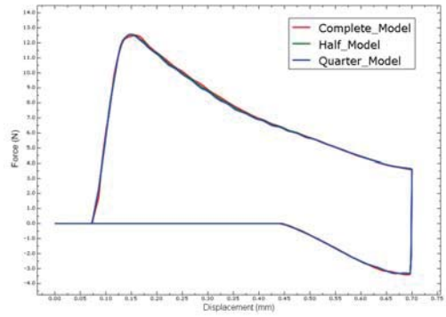
圖 6 完整模型與簡化模型之插拔力分析曲線
