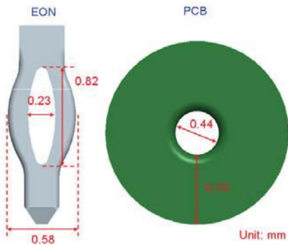
圖 3 針眼端子與 PCB 孔尺寸
